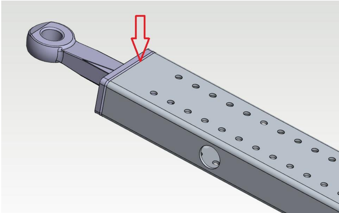
Kuva 2. Vetosilmän hitsiliitos
