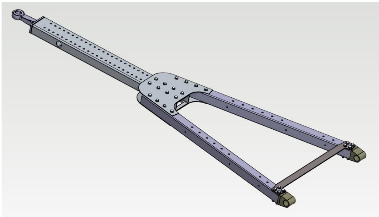
Kuva 1. M2017R vetoaisa
